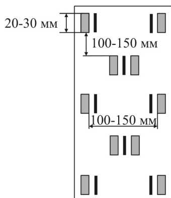
схема нанесения клея и скотча
