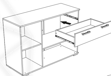
Рис.9 Установка выдвижного ящика
