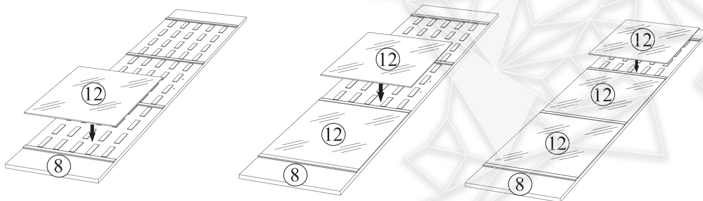
Рис.2 Схема наклейки зеркал на створку №8.
