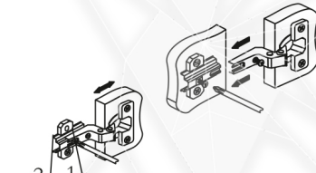
Регулировка створки по ширине
